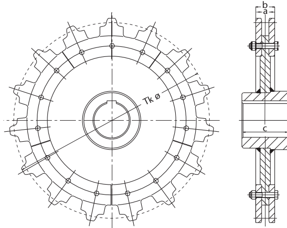
Abbildung 56: HEKO Kettenrad Typ GTA, taschenverzahnt, austauschbar, in geschweißter Ausführung
