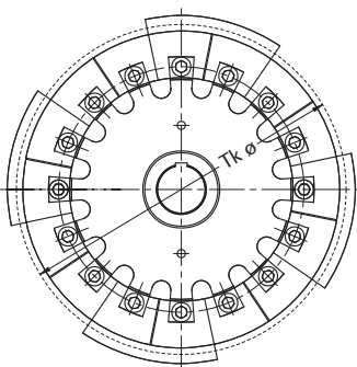
Abbildung 43: HEKOFLEX-Segment Typ RUHS mit gehärteten Kettenauflagen
