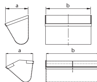
Abbildung 39: Hochleistungselevatorbecher und Mittenaustragungsbecher (v.o.n.u.)
