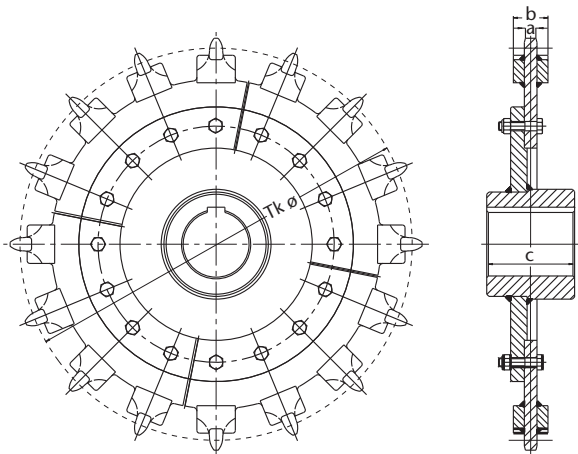
Abbildung 57: HEKO Kettenrad Typ GIA, innenverzahn- tes austauschbares Kettenrad mit ange- schweißter Kettenauflage
