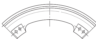
Abbildung 53: austauschbares 90° Segment für HEKO Kettenrad Typ RUP
