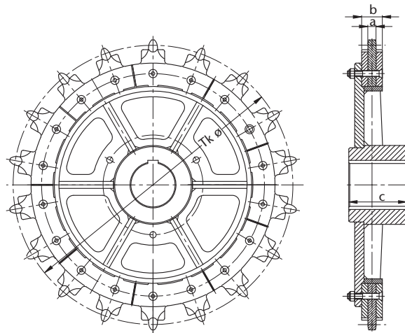
Abbildung 58: HEKO Kettenrad Typ GIA-3, innenverzahnt und austauschbar, für besonders hohe Anforderungen
