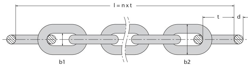
Abbildung 7: Maße für Rundstahlketten
