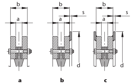
Abbildung 52 a: HEKO Kettenrad Typ RUP unverzahnt, austauschbar mit Stahlsegmenten Abbildung 52 b: HEKO Kettenrad Typ RUP I mit einseitigem Bordrand Abbildung 52 c: HEKO Kettenrad Typ RUP II mit beidseitigem Bordrand
