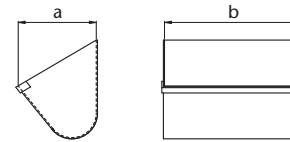
Abbildung 36: Becheraufbau B, mit vorderer Randverstärkung
