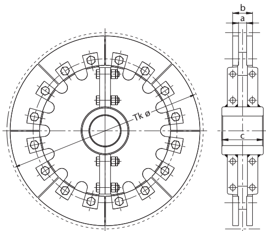
Abbildung 54: HEKO Kettenrad Typ RUG unverzahnt aus Stahl mit geteilter Stahlnabe
