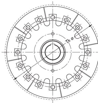
Abbildung 46a: HEKO Kettenrad Typ RUA unverzahnt, austauschbar mit Stahlsegmenten
