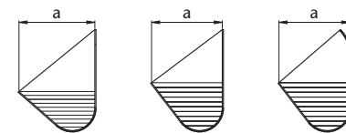
Abbildung 38: Elevatorbecher nach DIN 15233, DIN 15234, DIN 15235 (v.l.n.r.)
