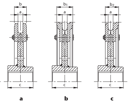
Abbildung 49b: HEKO Kettenrad Typ KS für Becher mit Rückwandbefestigung, mit beidseitigem Bordrand
