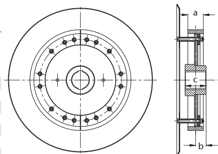
Abbildung 60: HEKO Umlenkrolle Typ BS, mit austauschbaren Lauftringen aus legiertem Sonderstahl
