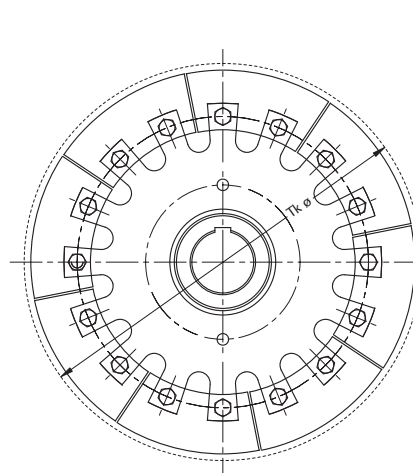
Abbildung 49a: HEKO Kettenrad Typ SUR für Becher mit Seiten- und Rückwandbefestigung, ohne Bordrand, Ausführungsbeispiel mit Stahlnabe
