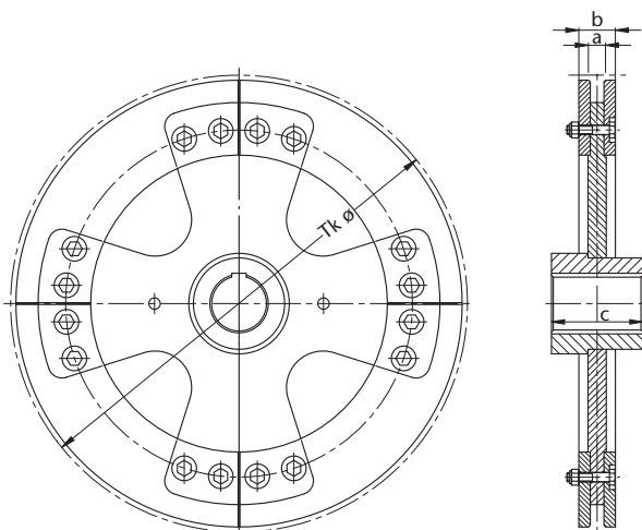
Abbildung 51: Kettenrad unverzahnt mit stahlsegmenten, austauschbar Typ RUR
