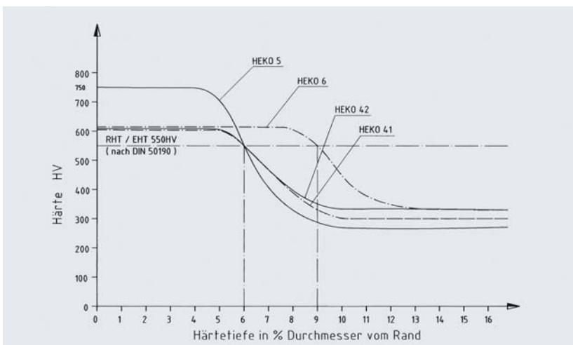
Abbildung 8: Härteverlaufskurven von Befestigungselementen aus Vergütungsstahl in gelenkgehärteter Ausführung sowie aus einsatzgehärteten Chrom-Nickel legierten Edeltählen
