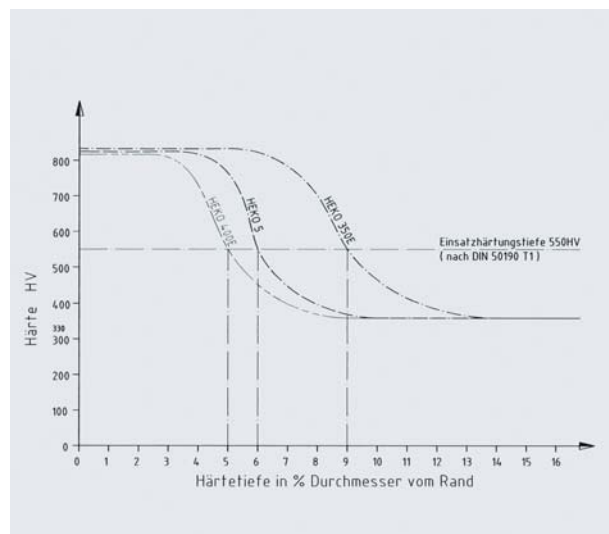
Abbildung 6: Härteverlaufskurven für HEKO Ketten aus Chrom-Nickel- bzw. Chrom-Nickel- Molybdän legierten Edeltählen
