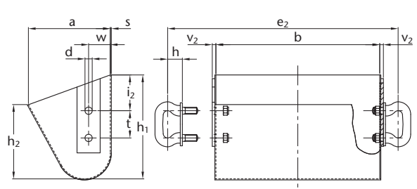
Abbildung 42: Becher gebohrt für Seitenbefestigung Form N
