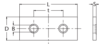
Abbildung 20: HEKO Distanzlasche für Kettenbügel Typ DIN 5699 und DIN 745
