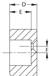
Abbildung 63: HEKO Lager-Buchse
