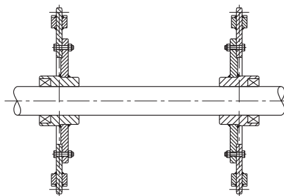
Abbildung 67: Montagehinweis
