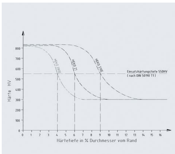
Abbildung 5: Härteverlaufskurven für HEKO Ketten aus Mangan-Kettensonderstählen
