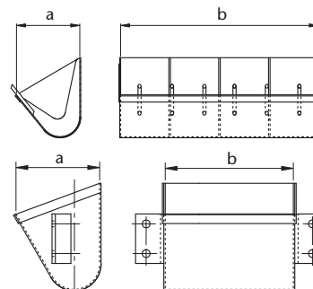
Abbildung 40: Bechersonderformen, Elevatorbecher mit Zähnen und Mittelsteg sowie Becher mit Befestigungswinkel (v.o.n.u.)
