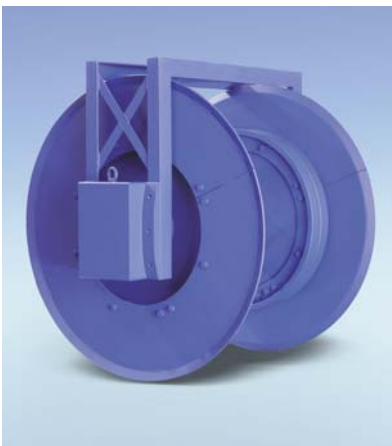
Abbildung 68: Vormontierte HEKO Umlenstation mit Segmentkettenrädern fixiert mit Zugankern
