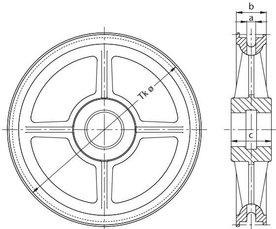
Abbildung 50: HEKO Kettenrad Typ GGB, einteilig und unverzahnt aus Grauguß
