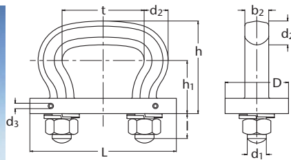
Abbildung 31: HEKO Kettenschloß Typ E
