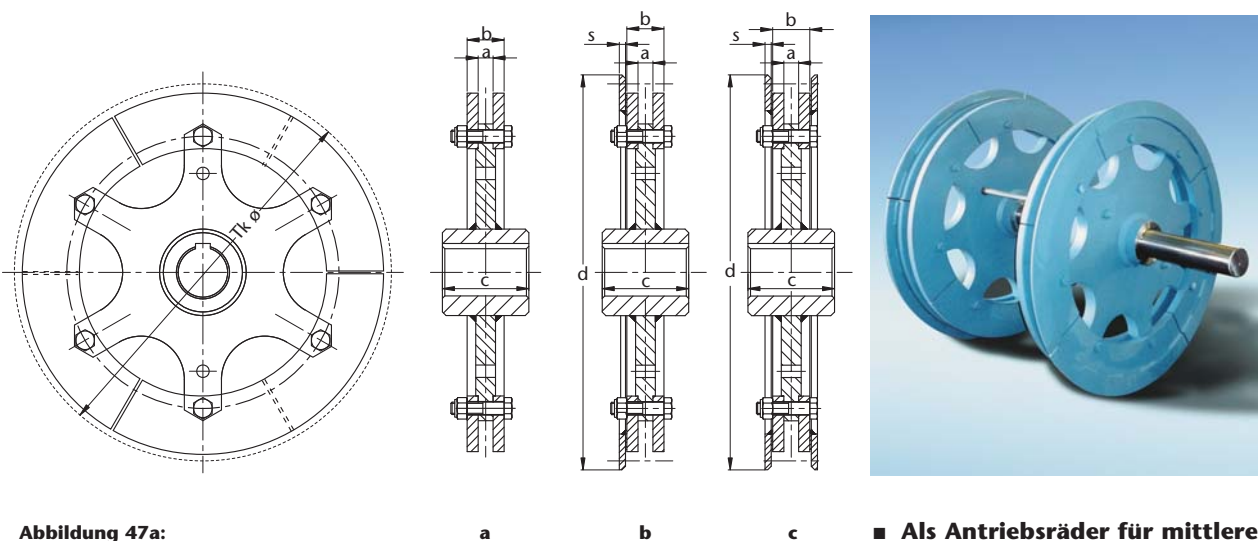
Abbildung 47a: HEKO Kettenrad Typ RUU unverzahnt, austauschbar mit Stahlsegmenten
