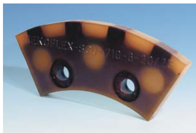
Abbildung 43: HEKOFLEX-Segment Typ RUHS mit gehärteten Kettenauflagen
