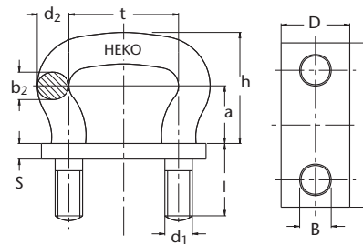
Abbildung 18: HEKO Kettenbügel Typ DIN 5699
