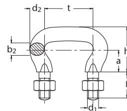
Abbildung 19: HEKO Kettenbügel Typ DIN 745
