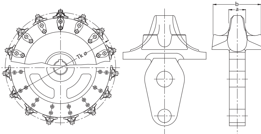
Abbildung 59: HEKO Kettenrad Typ RIS, innenverzahnt mit austauschbaren Einzelzähnen
