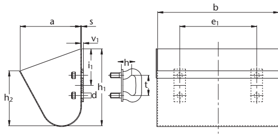
Abbildung 41: Becher gebohrt für Rückenbefestigung Form L
