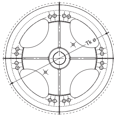
Abbildung 52: HEKO Kettenrad Typ RUP unverzahnt mit austauschbaren Stahlsegmenten
