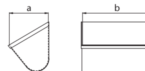
Abbildung 37: Becheraufbau C, mit dreiseitiger Randverstärkung
