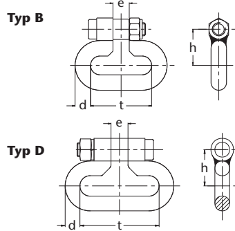
Abbildung 30: HEKO Kettenschloß Typ B mit angeschweißter Mutter, Typ D mit loser Mutter
