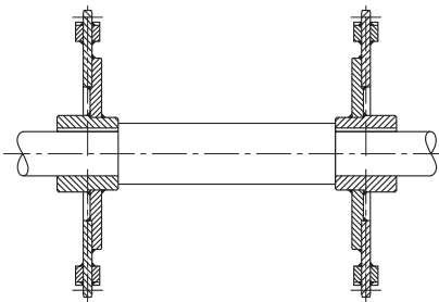
Abbildung 66: Montagehinweis
