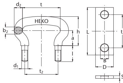
Abbildung 21: HEKO Kettenbügel Typ S
