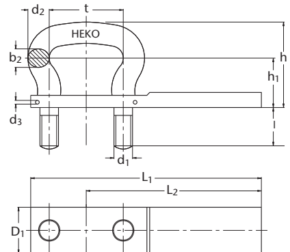
Abbildung 15: HEKO Kettenbügel Typ TS-L
